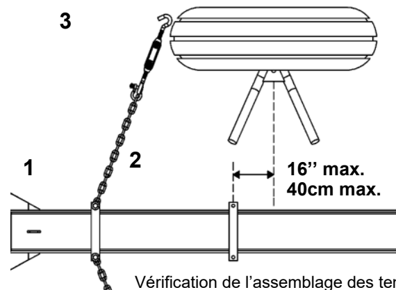
Vérification de l'assemblage des tendeurs
