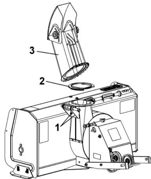
Installer goulotte
